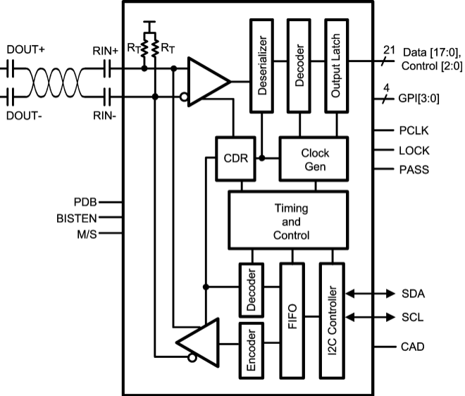
DS92LX2122 - DESERIALIZER
