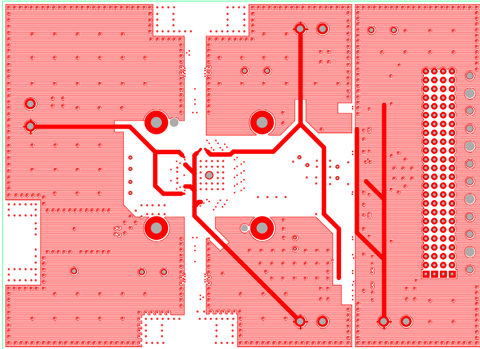
Layer 3: Power
