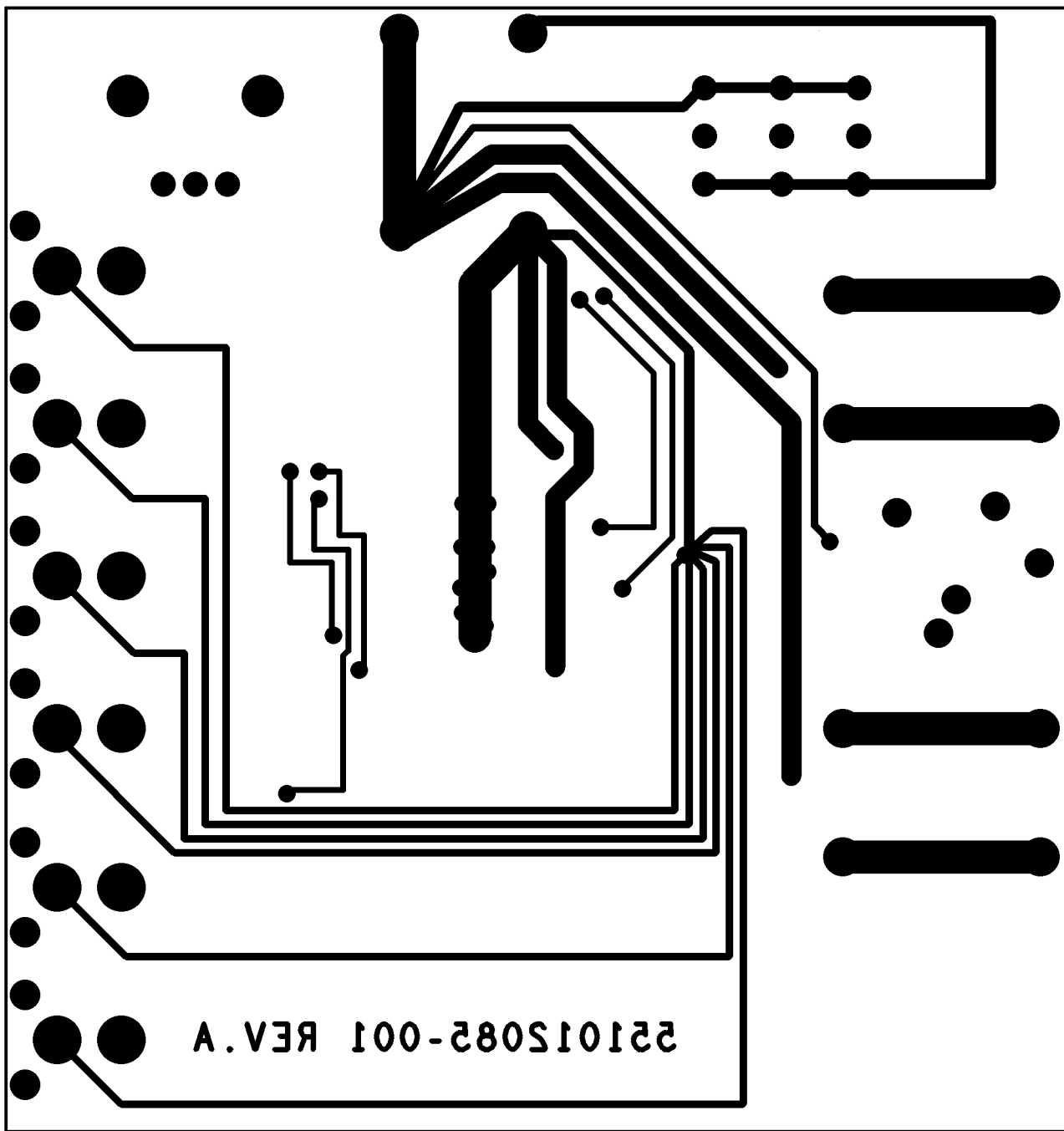
BOTTOM LAYER
