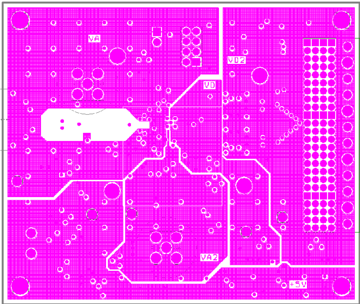
Layer 3 : Power
