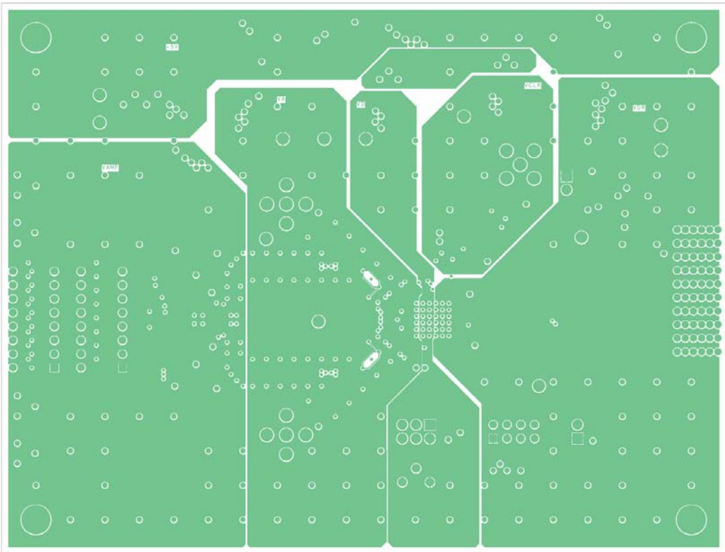
Layer 4 : Power
