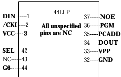
COP8Sxx7
