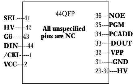
COP8Sxx7
