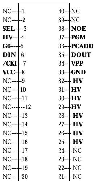
COP8Sxx7 40pin
