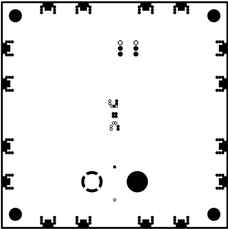
- LAYER 3 VCC PLANE
