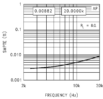
IMD 60 Hz, 4:1
