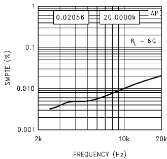
IMD 60 Hz, 1:1
