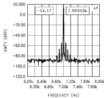
IMD 60 Hz, 7 kHz 1:1
