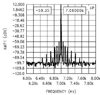
IMD 60 Hz, 7 kHz, 4:1
