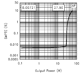
IMD 60 Hz, 7 kHz, 1:1
